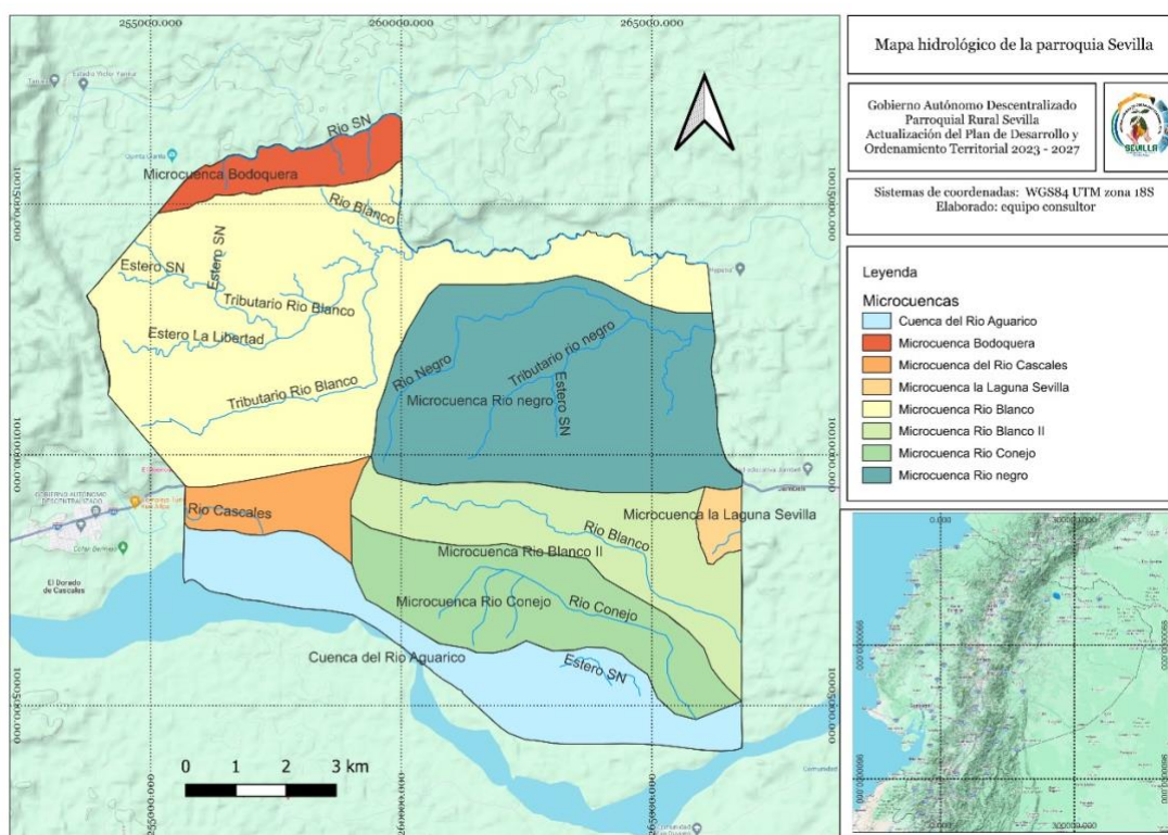
Figura 12. Mapa Hidrológico de Sevilla
