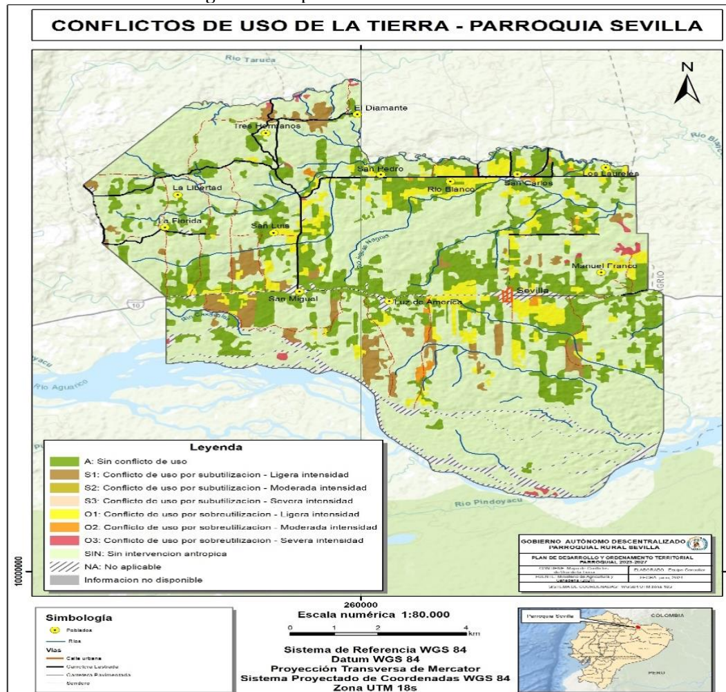
Figura 12. Mapa Conflictos de Uso del Suelo.
